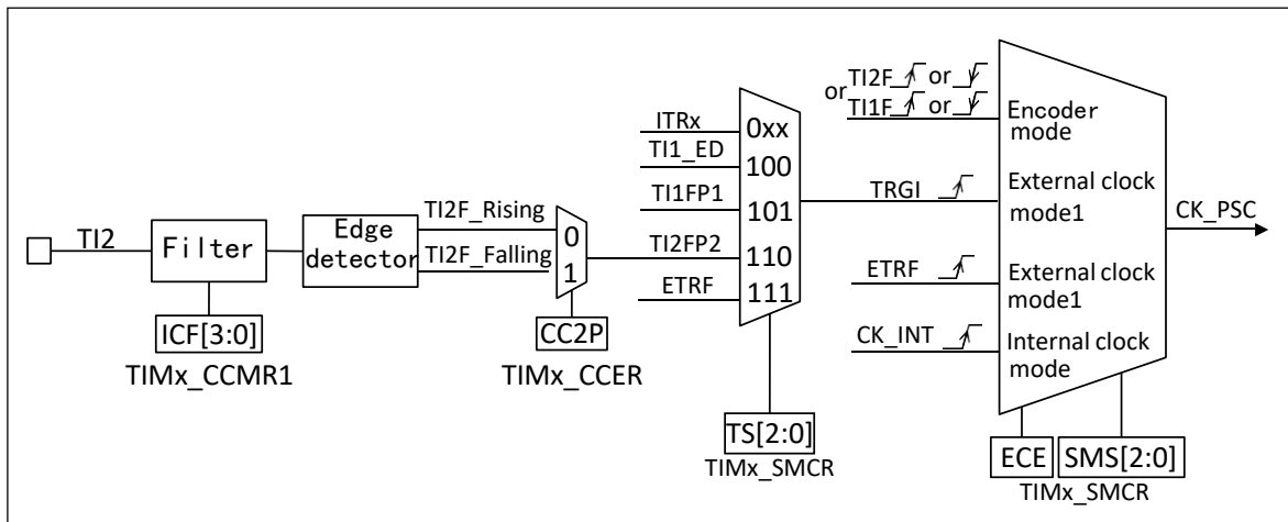
Fig 10.1-25 External trigger input module
