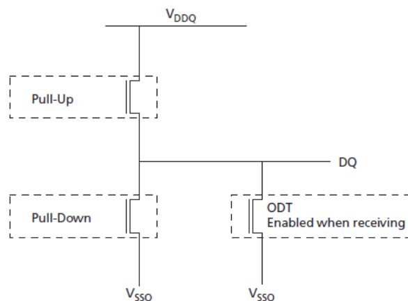
LVSTL I/O Cell
