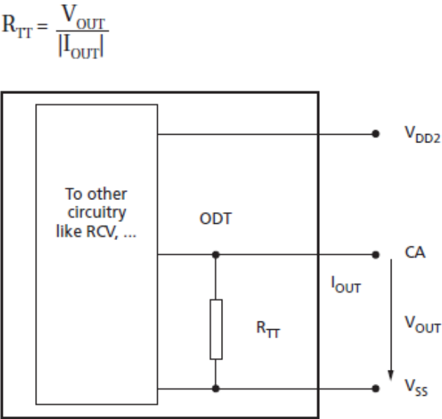
ODT for CA
