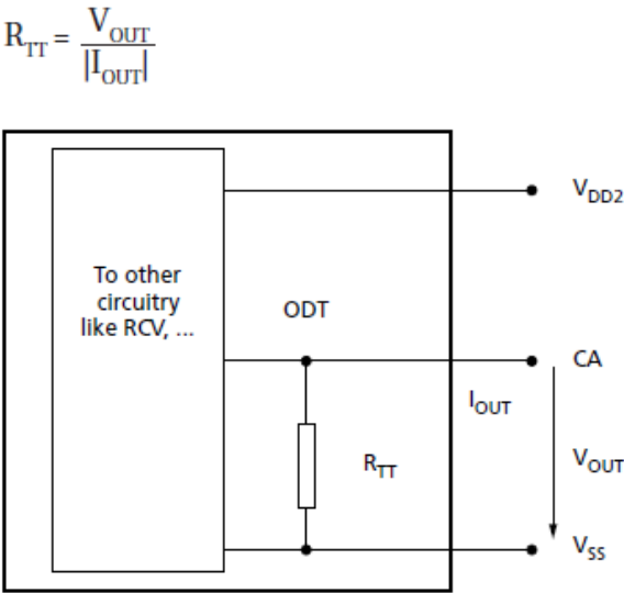
ODT for CA
