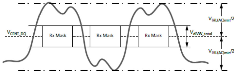
DQ V_{IHL(AC)} Definition (for Each Input Pulse)
