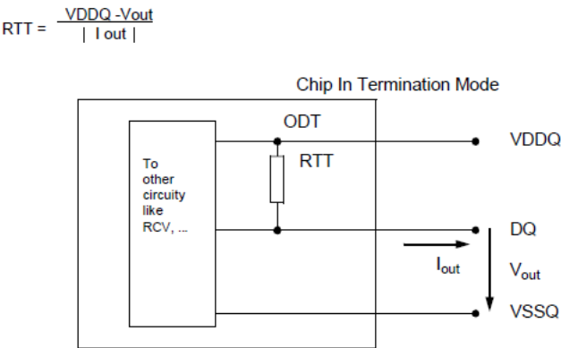
On Die Termination
