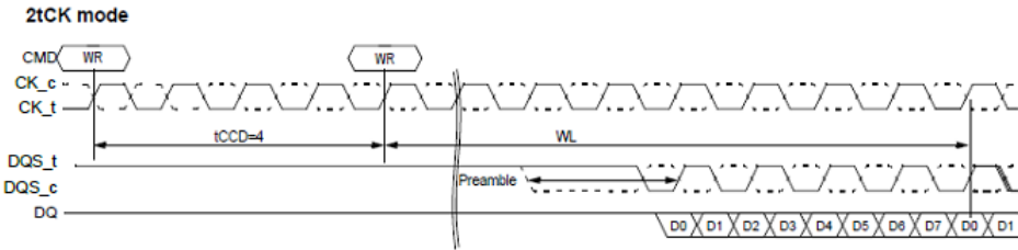
tCCD=4 (AL=PL=0)
