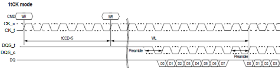
tCCD=5 (AL=PL=0)
