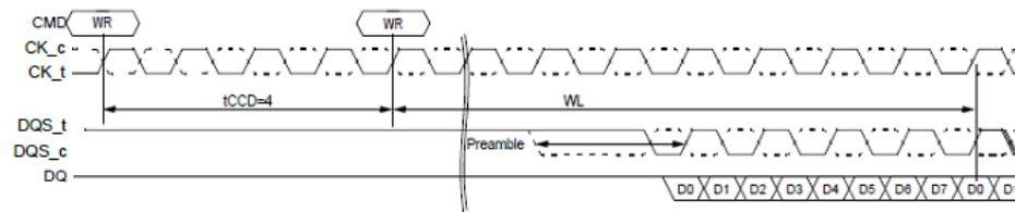
t_{CCD}=4 (AL=PL=0)
