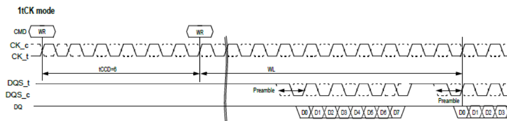
t_{CCD}=5 (AL=PL=0)
