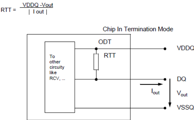
On Die Termination
