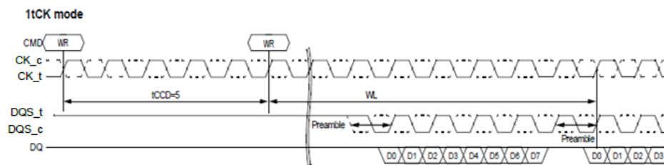
t_{CCD}=4 (AL=PL=0)
