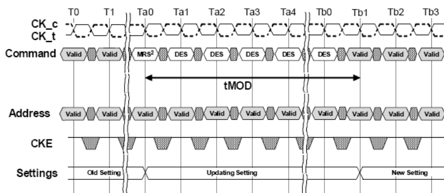
tMOD Timing
