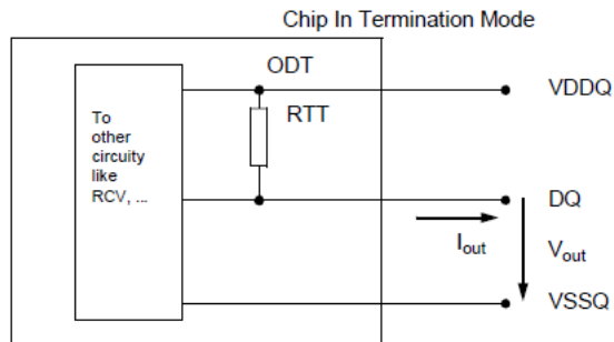
On Die Termination
